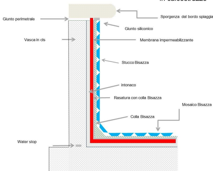
Sezione di una piscina tradizionale in calcestruzzo
